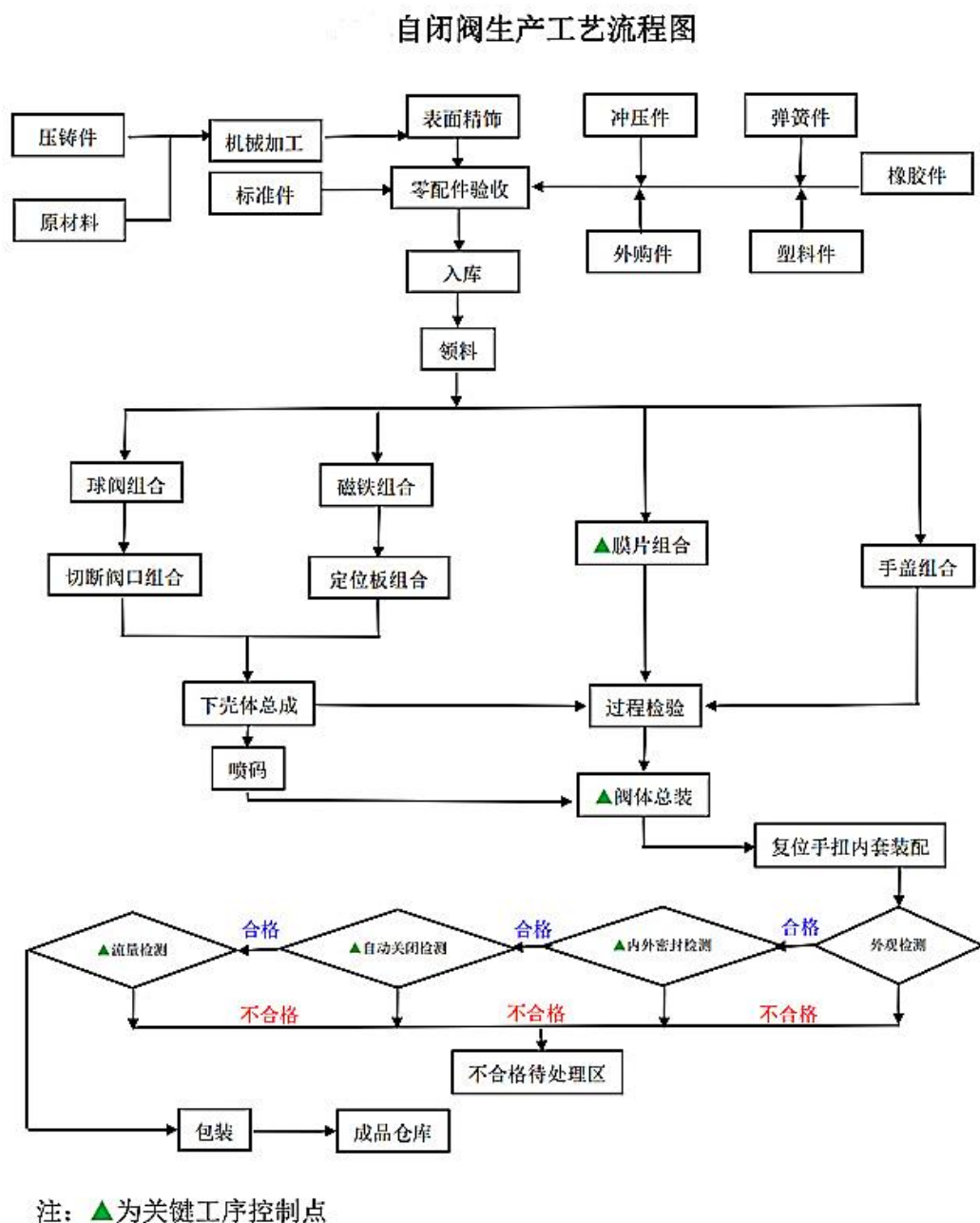
图 1 产品生产工艺流程图
